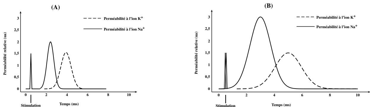
Figure 3 : Variation de la perméabilité de la membrane aux ions \text{Na}^+ et \text{K}^+ en en absence de DDT (A) et en présence de DDT (B)
