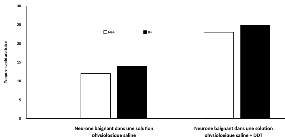
Figure 5 : Durée d'ouverture des canaux membranaires aux ions \text{Na}^+ et \text{K}^+ à la suite d'une stimulation
